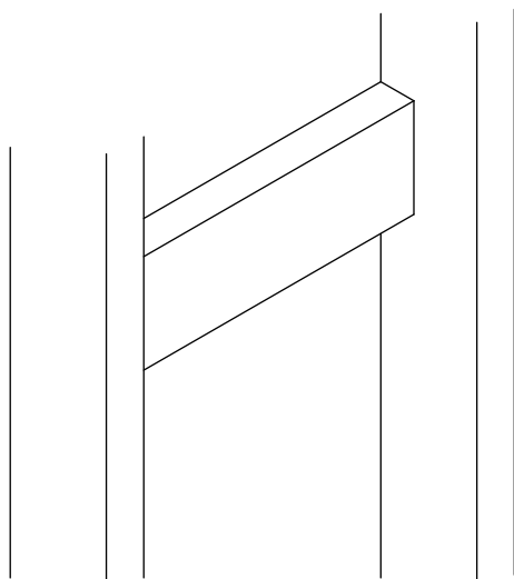
Espacement de montants 16 po (406 mm) standard
