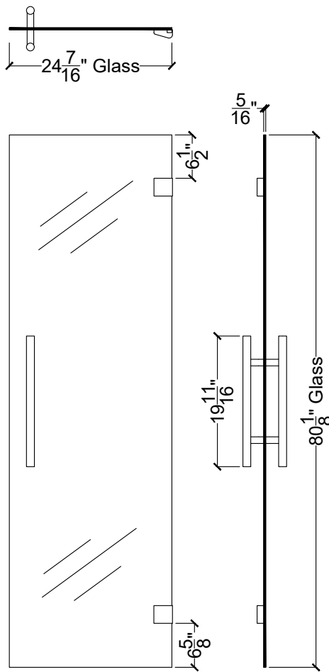
Door
