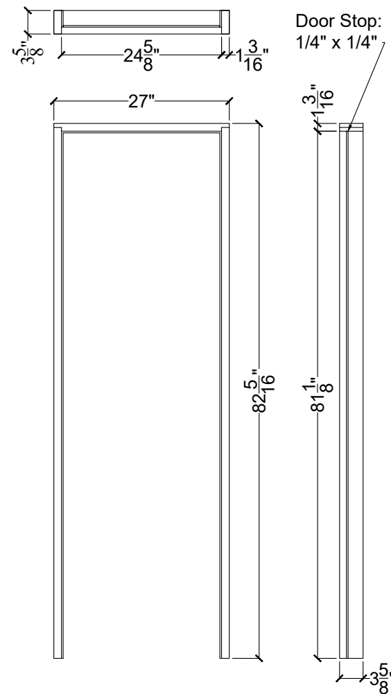
Door Jamb
