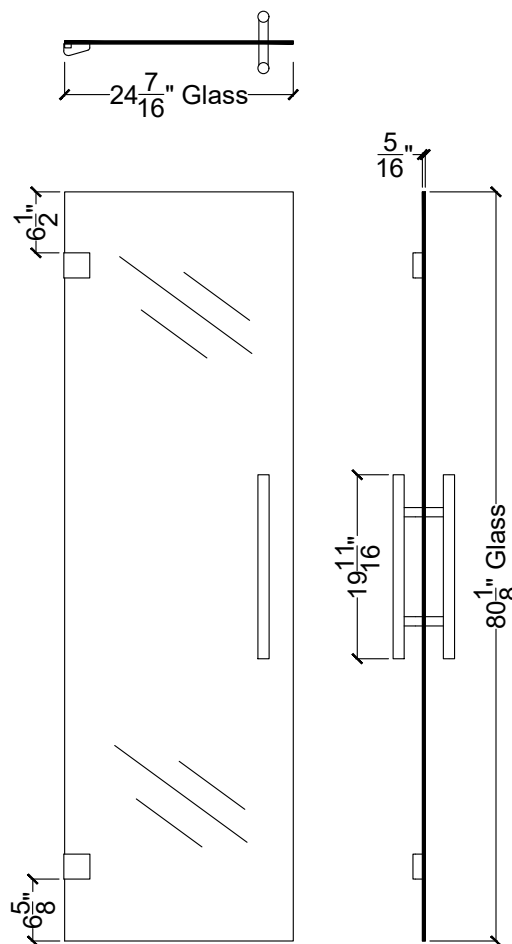
Door
