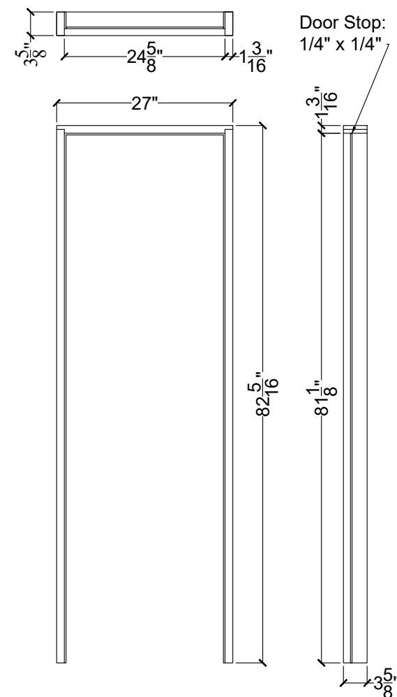
Door Jamb
