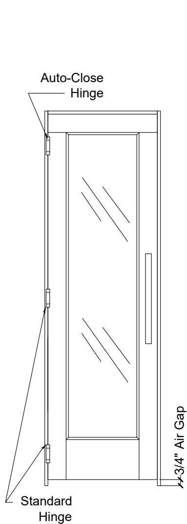
Door Assembly
