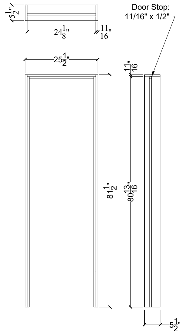
Door Jamb
