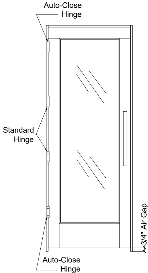
Door Assembly
