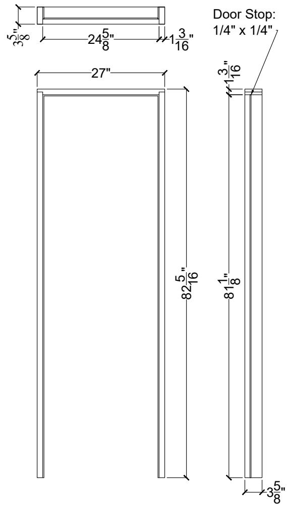
Door Jamb
