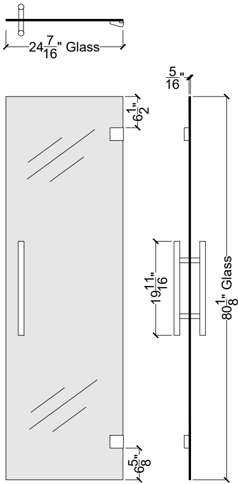
Door
