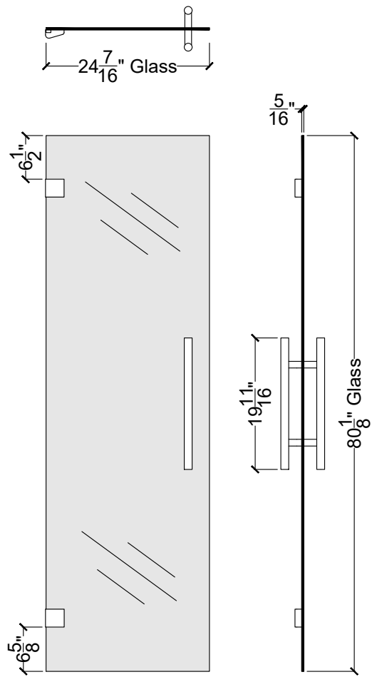
Door
