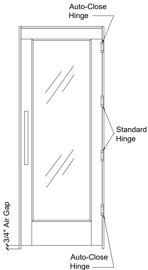
Door Assembly
