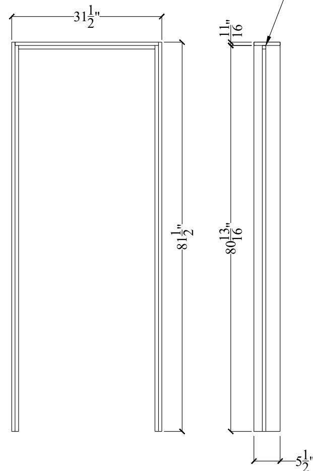
Door Jamb
